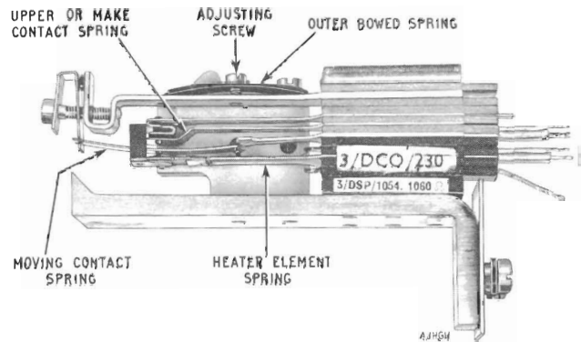
FIG. 2.—MARK 1A THERMAL SPRING-SET
